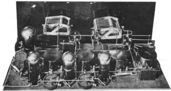
Een door Sarcos ontworpen 4-lamps raam-ontvanger met golfengte-transformatie, waarmede een buitengewoon hooge graad van selectiviteit bereikbaar is, zonder beïnvloeding van volume en toonkwaliteit. Deze ontvanger, de Sarcodyne, waarvoor de werkteekening gratis beschikbaar is gesteld, werd op de R.T.T. door de fa. Terwal geëxposeerd
