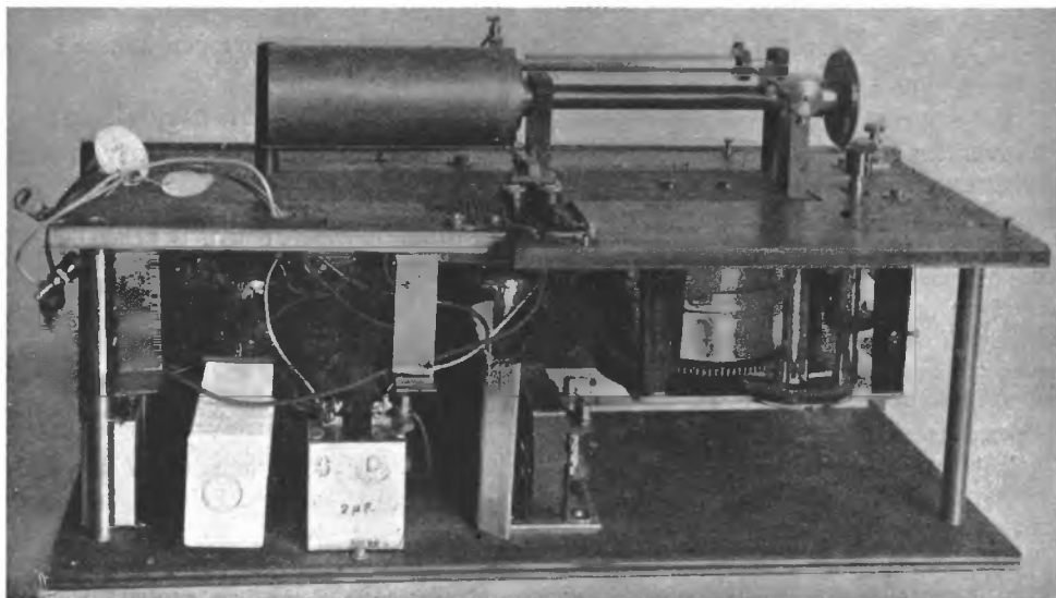
Foto van den uit zijn kast gelichten beeld-ontvanger. Duidelijker dan woorden toont deze wel aan, dat het voor de meerderheid onzer lezers onmogelijk zou zijn zonder hulp der radio-industrie zich een dusdanig apparaat te construeeren.
